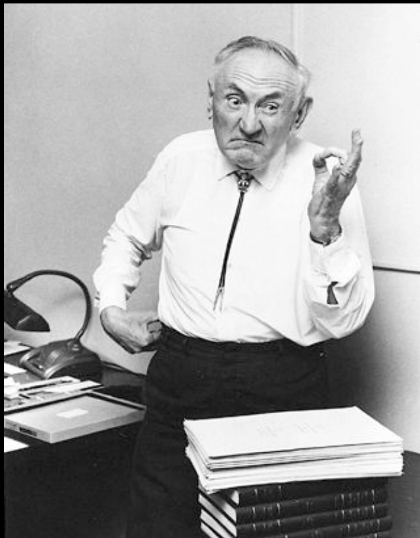
Fritz Zwicky
